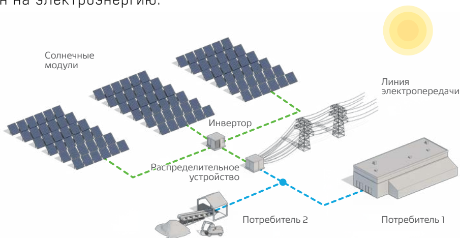
Схема организации работы солнечной электростанции параллельно с сетью
